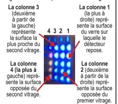
Figure 3: Réflexion provenant de 2 vitrages
